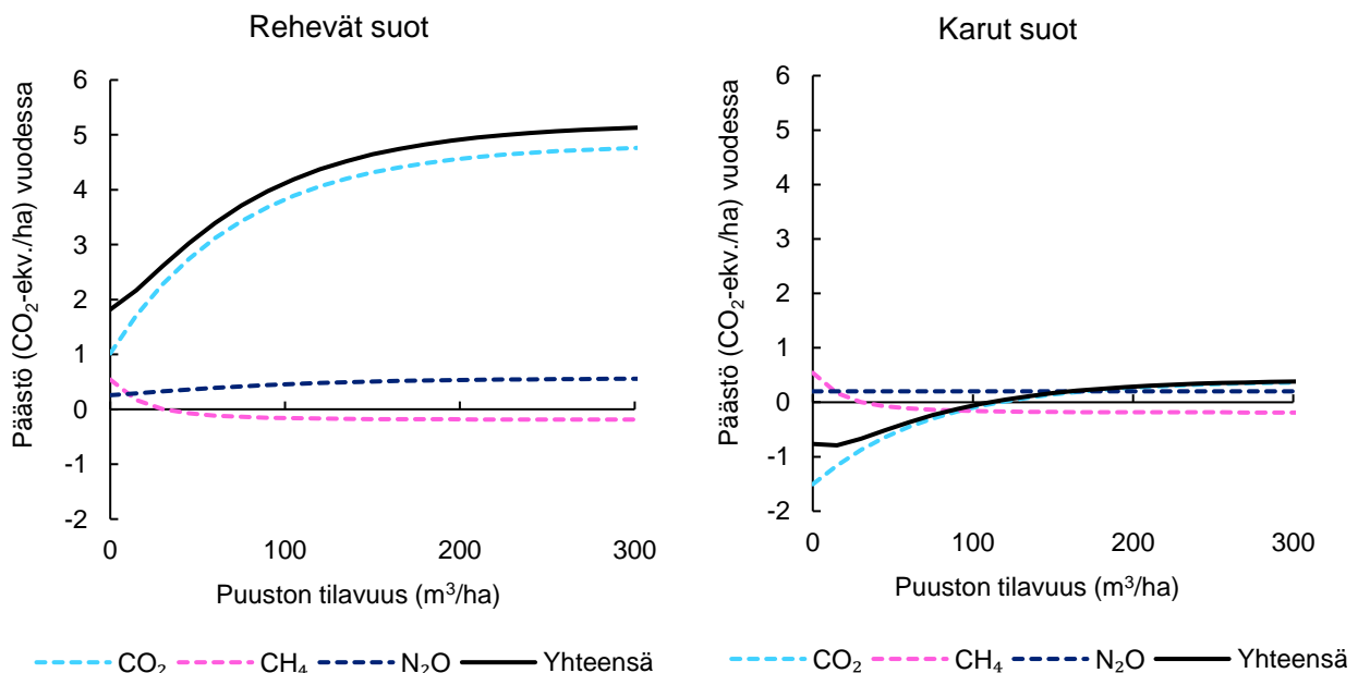
Kuva 2: Monsu-mallissa käytetyt kasvihuonekaasupäästöjen ja puuston tilavuuden väliset riippuvuudet ojitetulla suolla, kun leveysaste on 65°.
